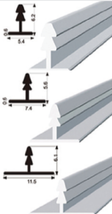
INLAY T PROFILE (FOR DÉCOR)
